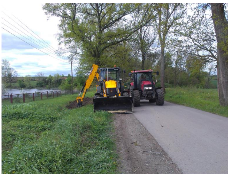
Poprawa odwodnienia jezdni- zbieranie zawyżonych poboczy i oczyszczanie rowów
